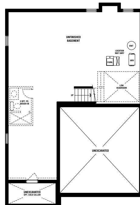
BASEMENT ELEV. 'A', 'B' & 'C'
